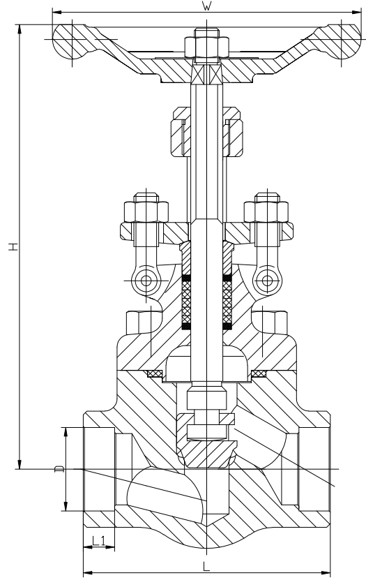
FGLV CLASS 800 ÖLÇÜLERİ (SW,BW,NPT)
