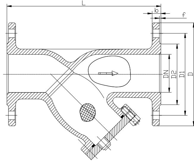
CSTR CLASS 150 ÖLÇÜLERİ(RF)
